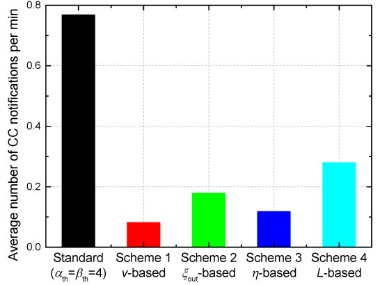
그림 10. 커버리지 클래스 변경 기법에 따른 단말의 분당 평균 커버리지 클래스 보고횟수 Fig. 10. The average number of coverage class notifications per min of each user according to the coverage class adaptation schemes
