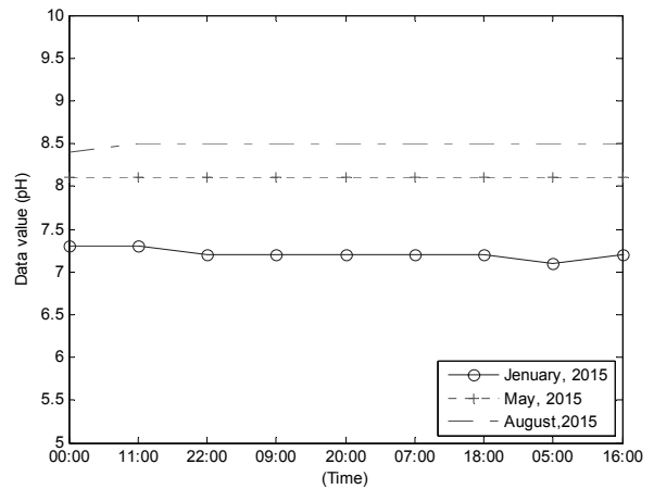
Fig. 20. Underwater pH
