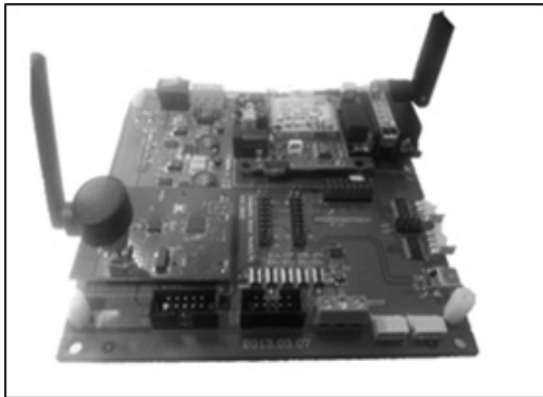
Fig. 14. Gateway[11]
