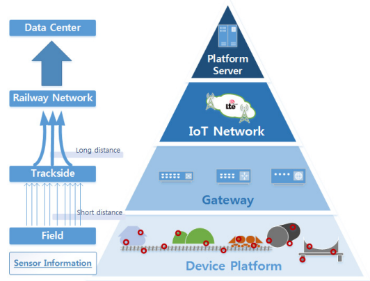
그림 3. 철도 환경에 적합한 IoT 플랫폼 구조 Fig. 3. The Architecture of IoT Platform in Railway Environment
