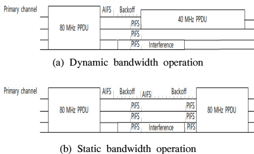
그림 1. Wi-Fi의 멀티채널 전송을 위한 대역폭 활용 방식 Fig. 1. Dynamic and static bandwidth operation for multi-channel transmission of Wi-Fi
