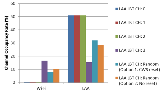
그림 4. LAA의 LBT 채널 방식에 따른 채널 점유율(Wi-Fi의 채널 분당 규칙을 LAA에 적용하지 않음)
