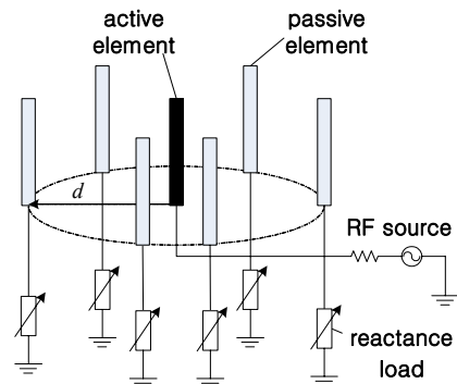
그림 1. SPA 안테나 구조 Fig. 1. SPA antenna structure
