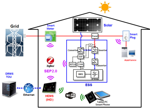
그림 1. 스마트 홈 구성도 Fig. 1. Smart Home Diagram
