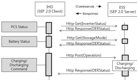
그림 2. SEP 메시지 흐름도 Fig. 2. SEP Message Flow
