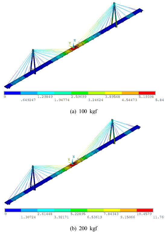
Fig. 6. ANSYS results
