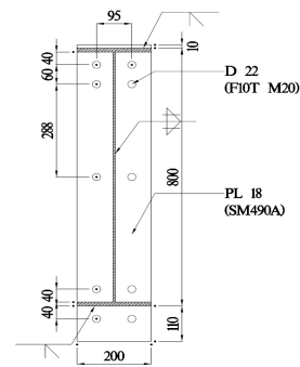
Fig. 5. End-plate detail
