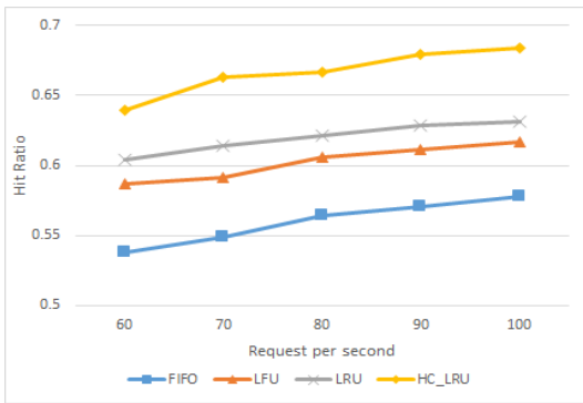
그림 11. 캐시정책에 따른 캐시 적중률 Fig. 11. Hit Ratio for Caching Policy
