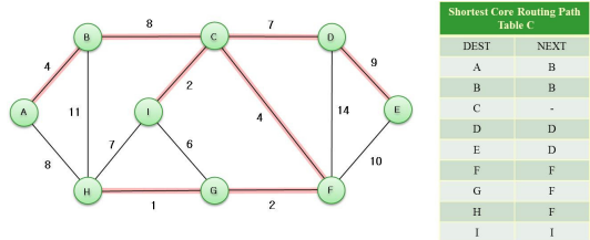
그림 4. SCRPT 테이블 Fig. 4. SCRPT Table
