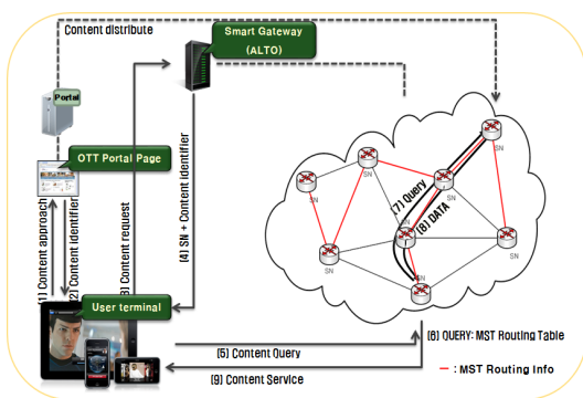
그림 1. 콘텐츠 전송 시나리오 Fig. 1. Contents Delivery Scenario
