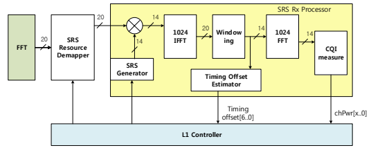
그림 7. 상향링크 사운딩 채널 수신부의 구조 Fig. 7. The uplink sounding channel receiver of Giga KOREA 5G.
