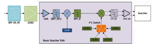
그림 11. Giga KOREA 5G 단말 동기 획득기의 RF부 인터페이스 Fig. 11. The RF interface for Giga KOREA 5G downlink time synchronizer.
