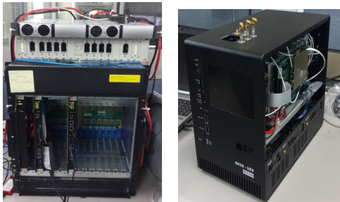
그림 14. Giga KOREA 5G 기지국 플랫폼(상)과 단말 플랫폼(하) 시제품 Fig. 14. The base station platform (left) and the mobile station platform (right) prototype
