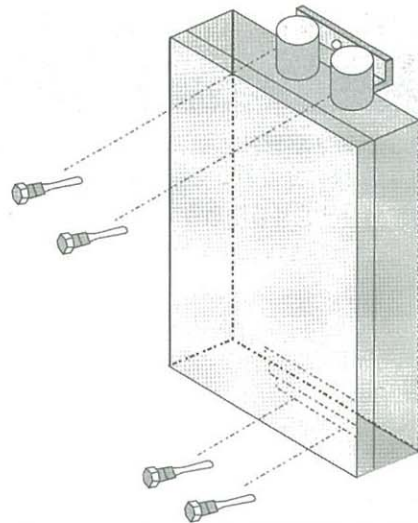
[ 벽걸이형 가스보일러를 앵커볼트로 설치한 예 ]
