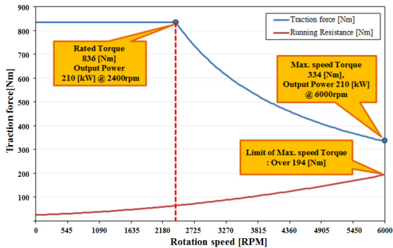
그림 1 도시철도차량용 IPMSM의 요구 견인력 곡선
