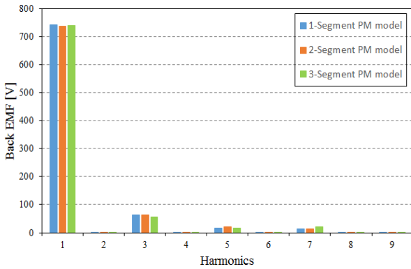
그림 5 정격속도 2400rpm에서 각 모델의 상 무부하 역기전력 고조파
