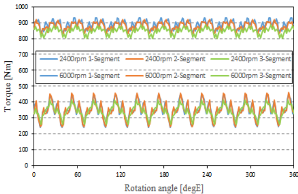
그림 3 각 모델의 정격, 최대 토크파형
