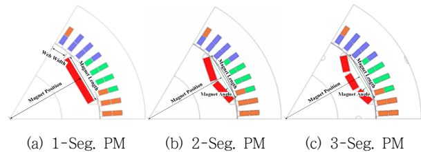
그림 2 Magnet segmentation에 따른 IPMSM 모델
