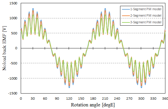
그림 4 정격속도 2400rpm에서 각 모델의 선간 무부하 역기전력 파형
