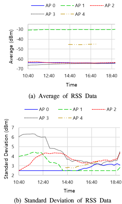
그림 4. 시간에 따른 근무지 위치 정보 그래프 Fig. 4. The time graph of workplace data
