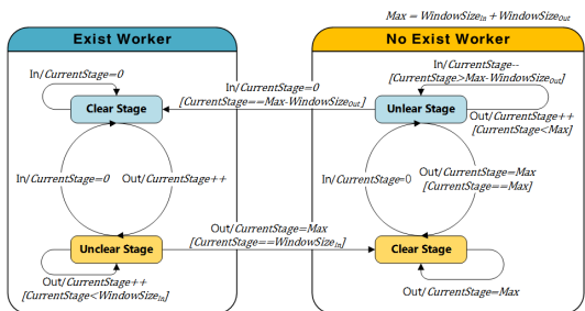
그림 2. 근무자가 위치하고 있는 근무지를 찾기 위한 상태 다이어그램 Fig. 2. The state diagram to detect a workplace which a worker is located.
