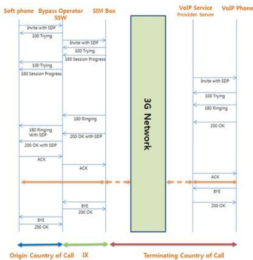
그림 4. SIM Box에 의한 Toll Bypass Fraud의 Call Flow Fig 4. Call Flow of Toll Bypass Fraud Using SIM Box
