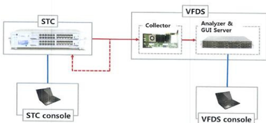
그림 7. SIM Box Detection System 의 10G급 트래픽 수집 및 처리 Test Bed 환경 Fig. 7. Test Bed of 10Gbps traffic collection & processing of SIM Box Detection System
