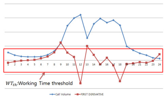
그림 6. 국내 24시간 Call Volume 과 업무 패턴 분석 예시 Fig. 6. Call Volume of operations around the clock & Analysis of working pattern
