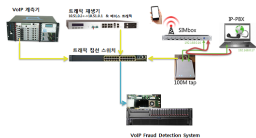
그림 8. SIM Box Detection System Test Bed 환경 Fig. 8. Test Bed of SIM Box Detection System
