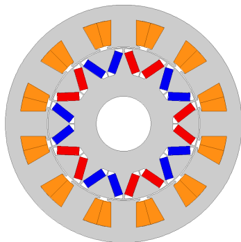
그림 2 해석을 위한 초기모델
