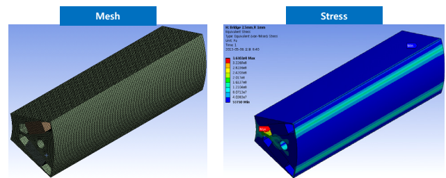
그림 4 초기모델의 응력해석 결과
