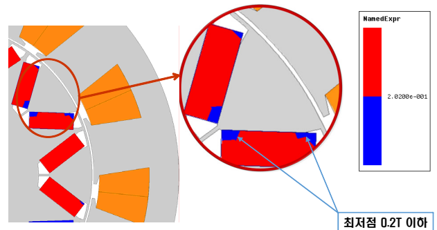
그림 3 초기모델의 감자해석 결과
