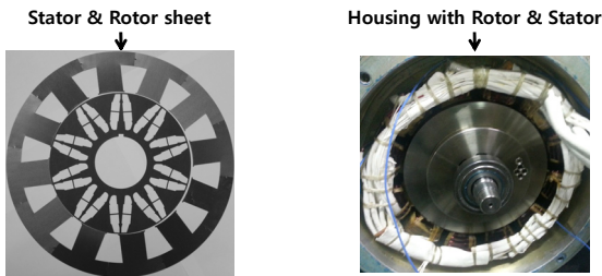
그림 12 제작된 모델 [9] Fig. 12 Manufactured model [9]
