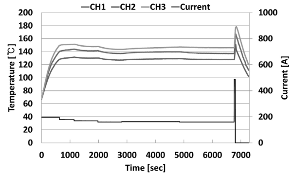
그림 15 온도포화를 고려한 최대부하 시험 결과 [9] Fig. 15 Maximum load test result considering the saturation temperature [9]
