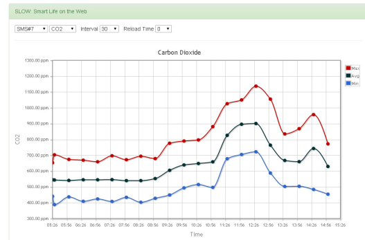
그림 7. 센서 데이터 화면 Fig. 7. Sensor data screen
