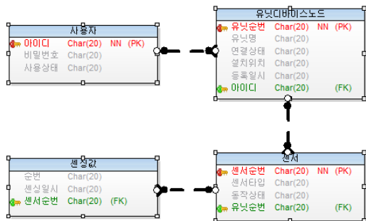
그림 4. ER 모델링 Fig. 4. ER Modeling
