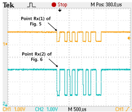
그림 11. 가시광 수신부의 포토다이오드 TSL-252r 측정 파형(그림 5의 Rx(1))과 LM358을 통해 9.2배 증폭된 파형(그림 6의 Rx(2)) Fig. 11. Output waveform at the photodiode TSL-252r and the OP amplifier IC LM358, i.e., Rx(1) and Rx(2) points.
