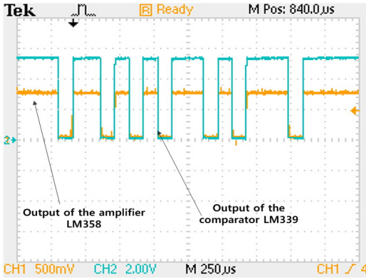
그림 15. 송수신 사이의 거리 300cm 에서의 LM358 증폭 파형과 LM339 비교기 출력 파형. Fig. 15. Output waveform at the comparator IC LM339 and the amplifier IC LM358 under the communication distance is 300cm.
