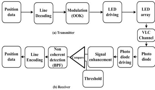
그림 2. 이 논문에서 제안한 거리 보상 기능이 포함된 문턱값 기반 가시광 통신 기법의 시스템 구조 Fig. 2. The system architecture of the threshold value based visible light communication built-in a distance compensation function proposed in this paper.
