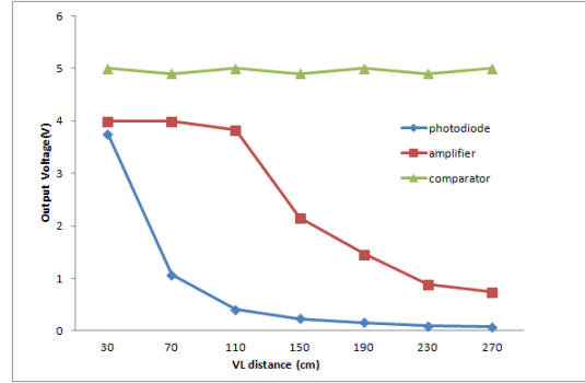
그림 16. 여러 가지 통신거리에 따라, 제안된 방식의 구현 프로토 타입에서 측정된 성능 비교 Fig. 16. Performance comparison in the proposed and implemented prototype depending on the communication distance.
