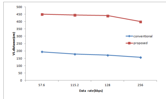
그림 17. 여러 가지 통신 시스템 속도에 따라, 제안된 가시광 통신 프로토 타입과 기존 방식사이의 통신거리 성능 비교 Fig. 17. Performance comparison of the proposed prototype and the conventional scheme depending on the communication speed.
