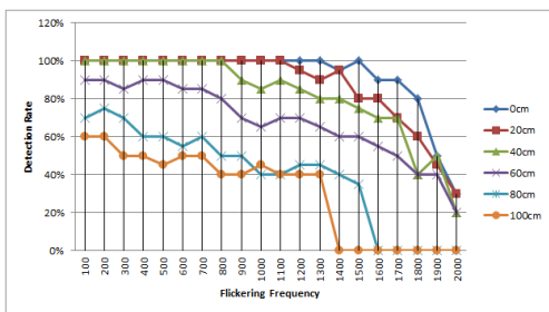
그림 13. 측정 거리에 따른 패턴 검출율 Fig. 13. Patten Detection Rate by Picturing Distance
