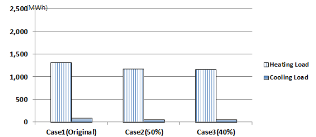
Fig. 3. Load graph(B)
