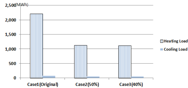
Fig. 4. Load graph(C)
