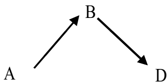
(전이성 인과-망)
