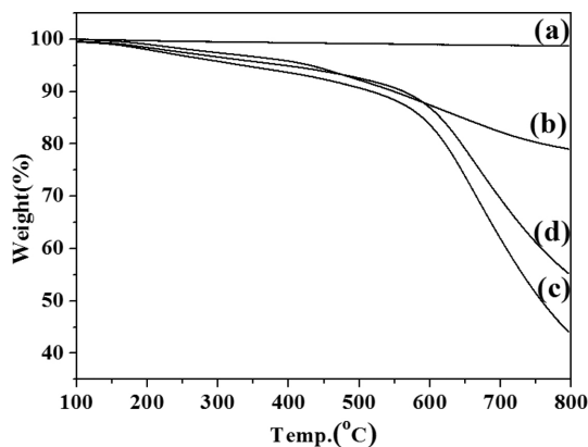
Fig. 2. TGA weight loss curves of (a) pristine MWCNT, (b) MWCNT-COOH(1), (c) MWCNT-COOH(2), and (d) MWCNT-COOH(3).
