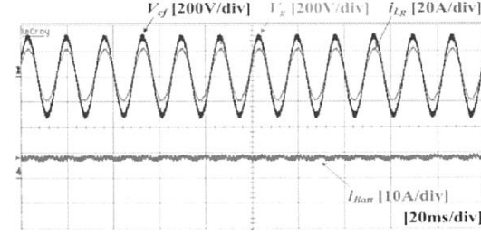
(d) Bi-directional inverter and battery current
