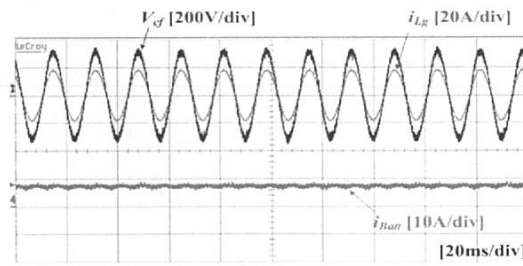
(d) Bi-directional inverter and battery current
