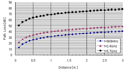
그림 4. ISM 대역 주파수의 실내 경로 손실 시뮬레이션 Fig. 4. Path loss simulation for ISM band indoor environment
