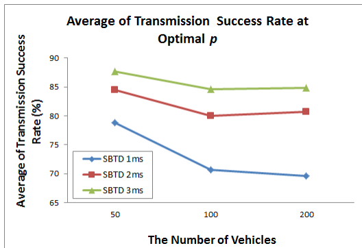
그림 10. 최상의 2차 릴레이 전송 확률 p 에서의 평균 전송 성공률 Fig. 10. Average of transmission success rate at optimal p
