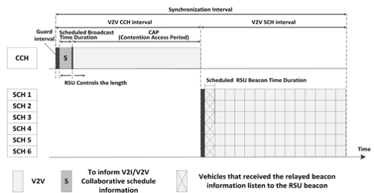
그림 3. V2V 프레임 및 멀티 채널 구조 Fig. 3. V2V frame and multi-channel architecture
