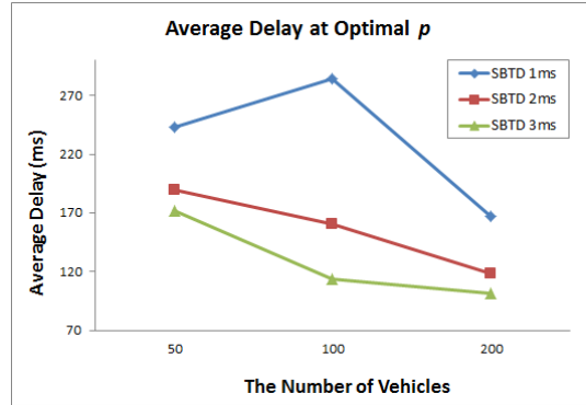
그림 11. 최상의 2차 릴레이 전송 확률 p 에서의 평균 지연 Fig. 11. Average delay at optimal p
