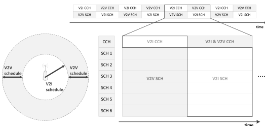
그림 1. V2I/V2V 영역과 V2I/V2V의 협력적 멀티 채널 구조 Fig. 1. V2I/V2V area and V2I/V2V collaborative multi-channel architecture
