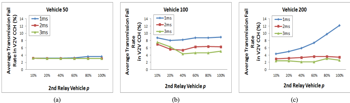
그림 8. 차량의 수가 50, 100, 200대인 경우, V2V 영역 안 차량의 평균 V2I/V2I 협력 메시지 전송 실패율 Fig. 8. Average transmission fail rate on different the number of vehicles
