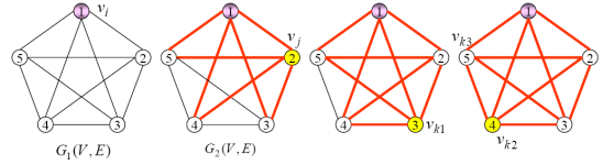
(d) G_4 graph 그림 3. MDVA 적용 결과 Fig. 3. Result of MDVA
