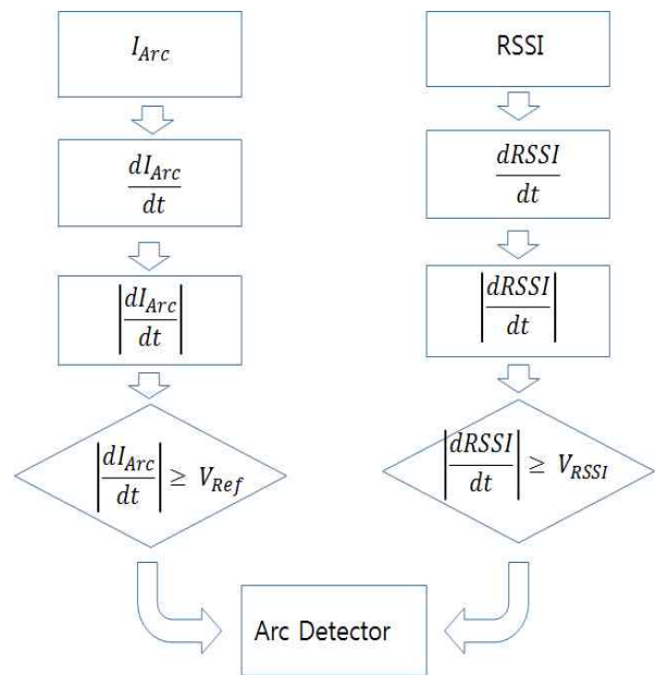
그림 5. 아크 신호의 신호처리 순서도 Fig. 5. Signal processing flow chart for arcing faults
