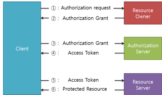
Fig. 1. OAuth protocol flow
