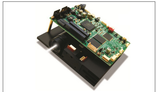
Fig. 6. DLP Module(DLP LightCrafter 4500 EVM)
