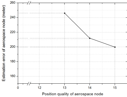
그림 6. 공중 노드 위치 품질에 따른 추정 오차 Fig. 6. Estimation error according to the position quality of aerospace node
