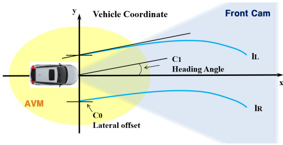
그림 2. 다항차수 기반 차선 모델 및 센서 인식 범위 Fig. 2. Lane model and sensor coverage.
