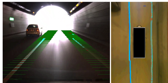
그림 6-b). 차선탐지 실험환경 (좌) 전방인식 (우)AVM인식
