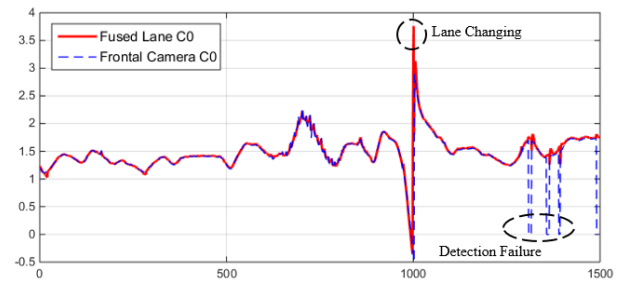
그림 6-a). 차선 융합 및 단일 차선의 Lateral Offset 비교
