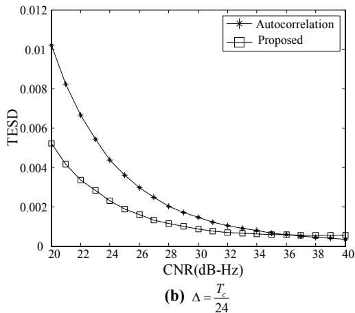
그림 5. 제안한 기법을 이용하였을 때와 자기상관함수를 이용하였을 때의 CNR에 따른 TESD 성능. Fig. 5. TESD performances of the proposed scheme and autocorrelation function as a function of CNR.
