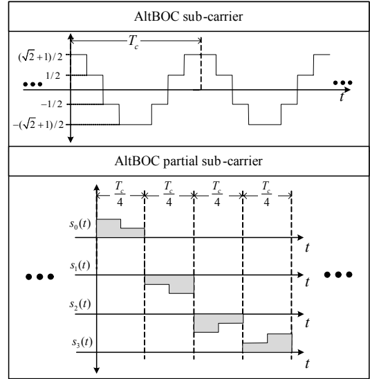
그림 1. AltBOC 신호의 부반송파와 부분 부반송파. Fig. 1. The AltBOC sub-carrier and partial sub-carriers.
