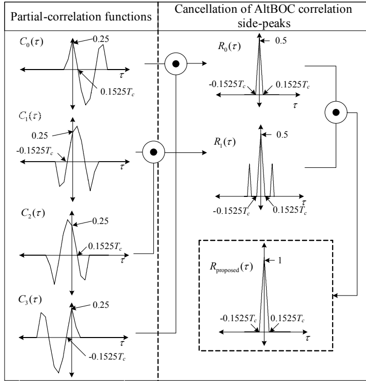
그림 4. AltBOC 신호의 부분 상관함수와 제안한 주변 첨두 제거 기법 Fig. 4. The partial-correlations of AltBOC signal and the proposed scheme of cancellation of AltBOC correlation side-peaks
