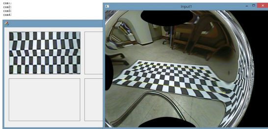
그림 8. 이미지 왜곡 보정 후 호모그래피를 이용하여 변환된 역원근 이미지 Fig. 8 After the distortion correction image by using the homography reverse perspective transformed screen
