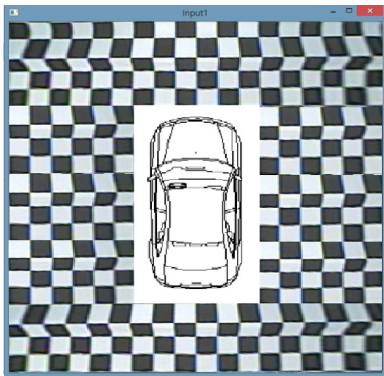
그림 9. 4개의 영상을 한 개의 영상으로 합친 이미지 Fig. 9 After the distortion correction image by using the homography reverse perspective transformed screen
