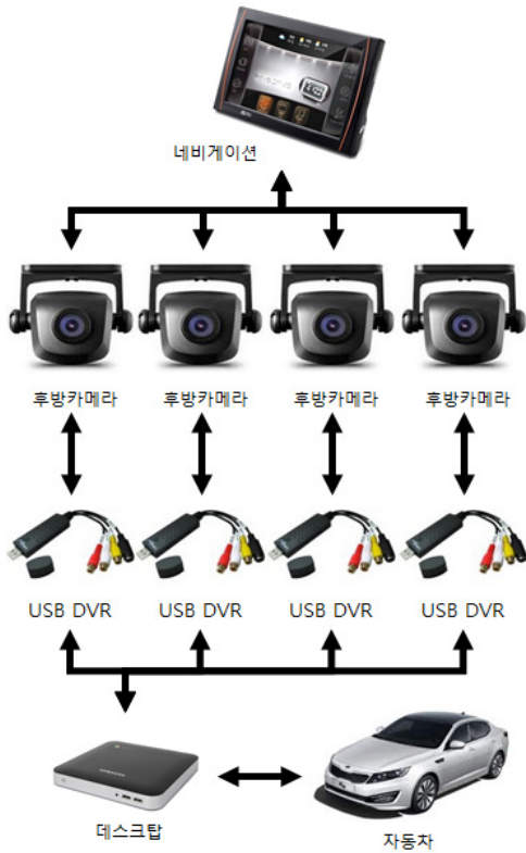
그림 5. 시스템 구조 Fig. 5 System structure
