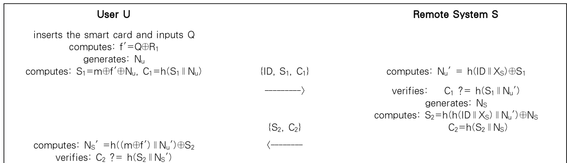
그림 1. An의 로그인 단계와 인증 단계 Fig. 1. An' Login Phase and Authentication Phase
