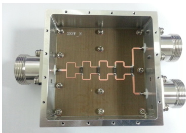
그림 3. 제작한 Wilkinson 전력분배기 사진
