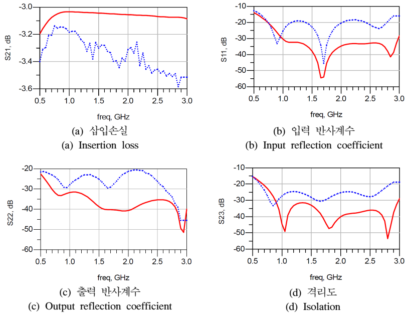
그림 1. 광대역 분배기의 성능 시뮬레이션 및 측정 결과(시뮬레이션 :실선, 측정 :점선)
