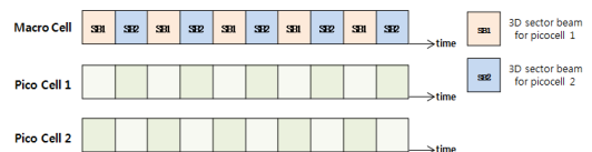
그림 4. 제안하는 셀간 간섭 제어 기법 예시 Fig. 4. An example of proposed inter-cell interference coordination
