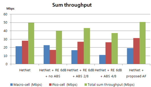
그림 8. 매크로 셀과 피코 셀의 수율 합
