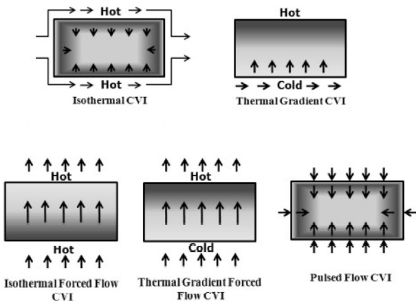
Fig. 3. CVI techniques
