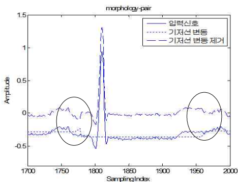
그림 8. morphology-pair 연산으로 기저선 변동을 제거 Fig. 8. Eliminate baseline drift by the morphology-pair operation
