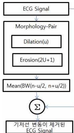
그림 9. 제안한 기저선 변동 잡음 제거 알고리즘의 흐름도 Fig. 9. Proposed flowchart for elimination of ECG baseline variation noise.
