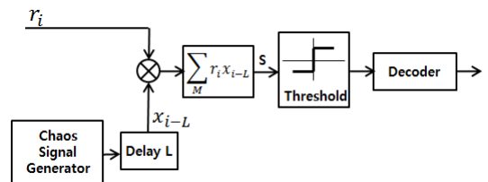
그림 4. 제안한 카오스 수신기. Fig. 4. Proposed chaos receiver.
