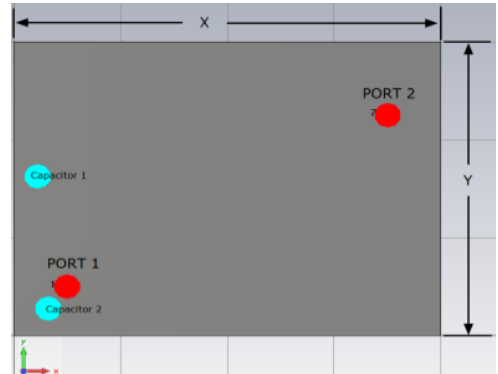
그림 6. 디커플링 캐패시터의 용량 및 위치결정 Fig. 6 Positioning and capacity of the decoupling capacitor
