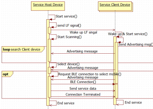
그림 3. 저주파를 이용한 이웃하는 단말간 기회기반 컴퓨팅 서비스 순서 다이어그램 Fig. 3. Sequence diagram of B-PniP that use Low Frequency
