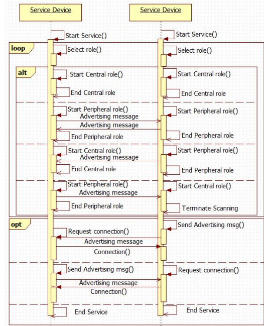
그림 5. 블루투스 저에너지 프로토콜 단말 역할 변경을 통한 기회기반 서비스 역할 결정을 위한 과정 Fig. 5. Process for determining B-PniP service role using role switching
