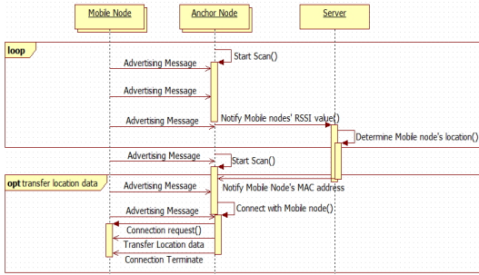
그림 2. 실제 위치인지 프로토콜 순서 다이어그램 Fig. 2. Sequence diagram of B-LIDx protocol
