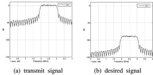
Fig. 3. Spectrum of transmit signal and received desired signal in own station 그림 3. 자국의 송신 신호와 수신 신호의 신호 전력 스펙트럼
