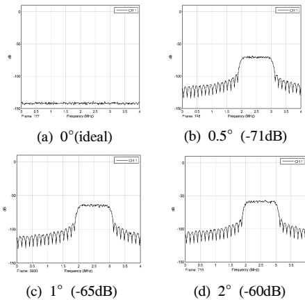
Fig. 5. Spectrum of self-interference signal after RF cancellation according to phase shifter error 그림 5. 위상 천이기 오차에 따른 RF Cancellation 후에 남은 자기 간섭 신호 스펙트럼
