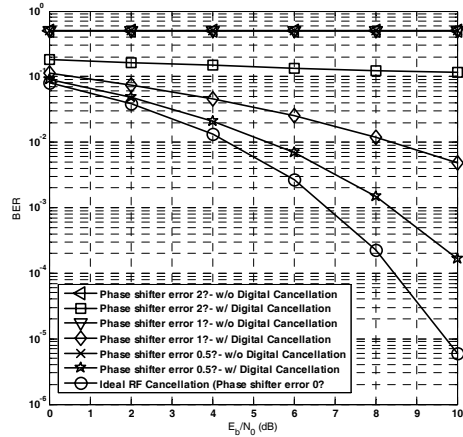
Fig. 7. BER performance of SSD system according to phase shifter error 그림 7. 위상 천이기에 오차에 따른 SSD 시스템의 성능
