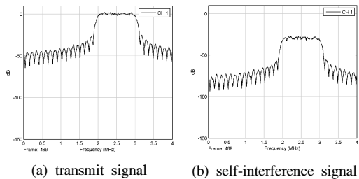
Fig. 4. Spectrum of transmit signal and direct self-interference signal of own station 그림 4. 자국의 송신 신호와 직접 자기 간섭 신호의 전력 스펙트럼
