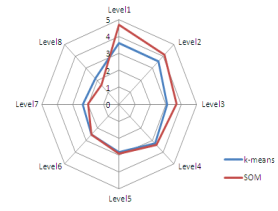
그림 4. 고객수준별 평균요스값 비교
