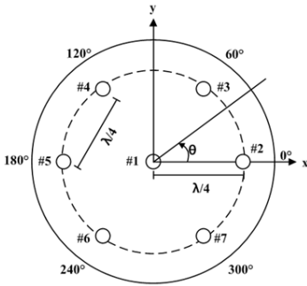
그림 2. 7소자 ESPAR 안테나의 구조 Fig. 2. Structure of 7-element ESPAR antenna
