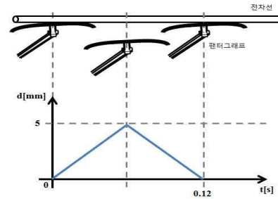
그림 8. 이선현상의 개념도 Fig. 8. The schematic of pantograph detachment
