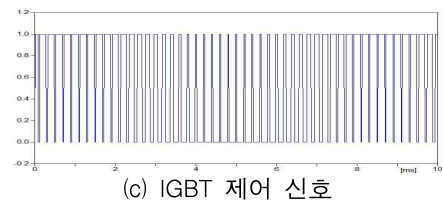
그림 7. IGBT 모듈 입력신호 Fig. 7. The input signal to IGBT module
