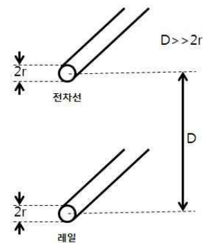
그림 3. 전차선과 레일 Fig. 3. The catenary wire and rail
