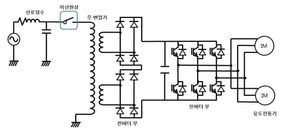
그림 2. 전체 집전시스템 모델링 개략도 Fig. 2. The schematics of whole electric feeding system model
