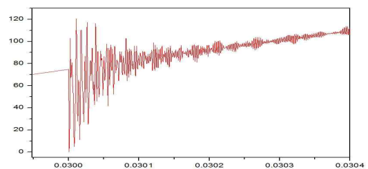
그림 10. 이선아크 파형 Fig. 10. The waveform of pantograph detachment arc
