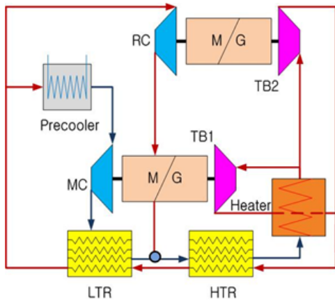
Fig. 7 샌디아 국립연구소 시험장치 개념도
