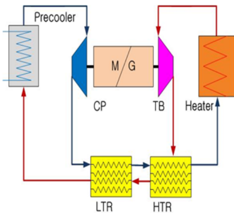
Fig. 9 일본 에너지연구소 시험장치 개념도
