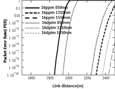
그림 8. \lambda=850\text{nm} , 1310\text{nm} , 1550\text{nm} 에 대한 16-DPIM과 16-PPM 방식의 PER 비교 Fig. 8. 16-DPIM and 16-PPM PER for \lambda=850\text{nm} , 1310\text{nm} and 1550\text{nm} .
