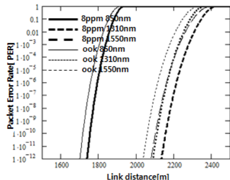
그림 4. \lambda=850nm, 1310nm, 1550nm 에 대한 8-PPM과 OOK 방식의 PER 비교 Fig. 4. 8-PPM and OOK PER for \lambda=850nm, 1310nm and 1550nm.
