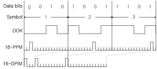
그림 1. 데이터 비트와 전송되는 심벌 OOK, 16-PPM과 16-DPIM Fig. 1. Mapping of data bits to transmitted symbols for OOK, 16-PPM and 16DPIM
