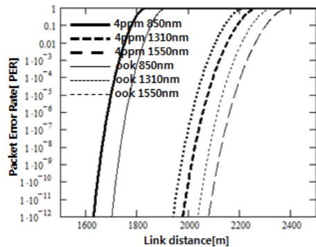
그림 3. \lambda=850nm, 1310nm, 1550nm 에 대한 4-PPM 과 OOK 방식의 PER 비교 Fig. 3. 4-PPM and OOK PER for \lambda=850nm, 1310nm and 1550nm.
