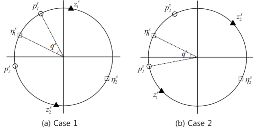
그림 3. 단위 원 위의 상관값의 위치 Fig. 3. Position of the correlation value on the unit circle
