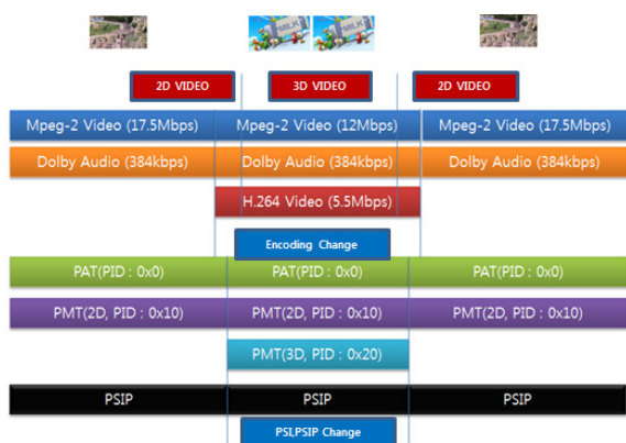
그림 5. 시간에 따른 Transport Stream 구성 Fig. 5. Construction of Transport Stream in time
