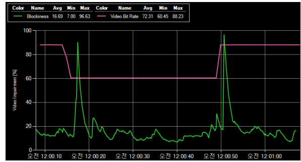
그림 3. ASI 신호 스위칭 시 분석 화면 Fig. 3. Analysis screen in switching ASI
