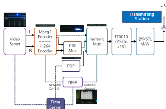
그림 6. Seamless 전환용 3D 송출시스템 Fig. 6. Headend system of switching 2D and 3D seamlessly
