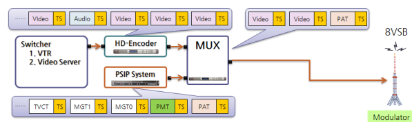
그림 9. DTV 송출 시스템 구성 Fig. 9. Composition of DTV Head-End System
