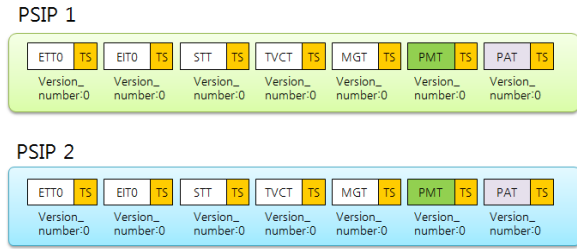
그림 10. 2개의 PSIP 테이블의 version_number 값이 같을 경우의 예시 Fig. 10. Example of the same version_number about PSIP Table
