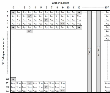
그림 1. 동기변조 방식에서의 OFDM 세그먼트 구조 Fig. 1. OFDM Segment configuration for synchronous modulation
