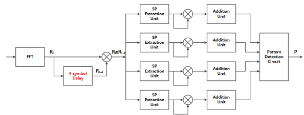
그림 3. 제안한 분산 파일럿 위치 추정 방법 Fig. 3. Proposed SP Position Estimation Method
