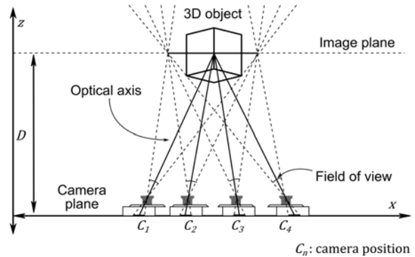
그림 1. Recentering camera 방식의 원근 투영 이미지 획득. Fig. 1. Acquiring perspective images by using recentering camera method.
